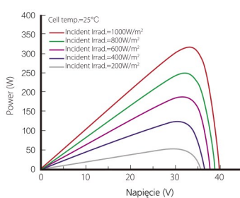
Wykres moc-napięcie
